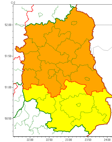
Silny wiatr 2022-05-21 05:49
