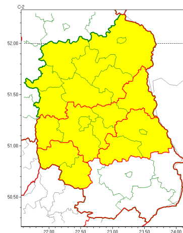
Opady śniegu 2022-04-01 22:58
