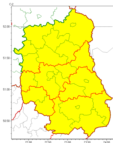
Oblodzenie 2022-04-01 22:58
